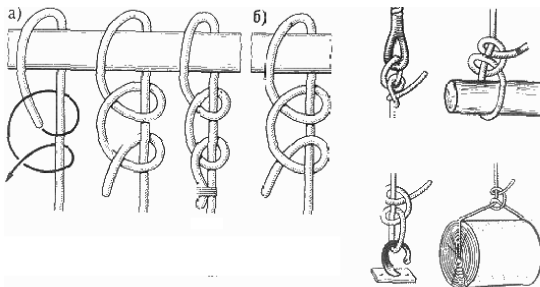
А Рис. 10. Простой штык: а - правильно завязанный; б - перевернутый (неправильный)
