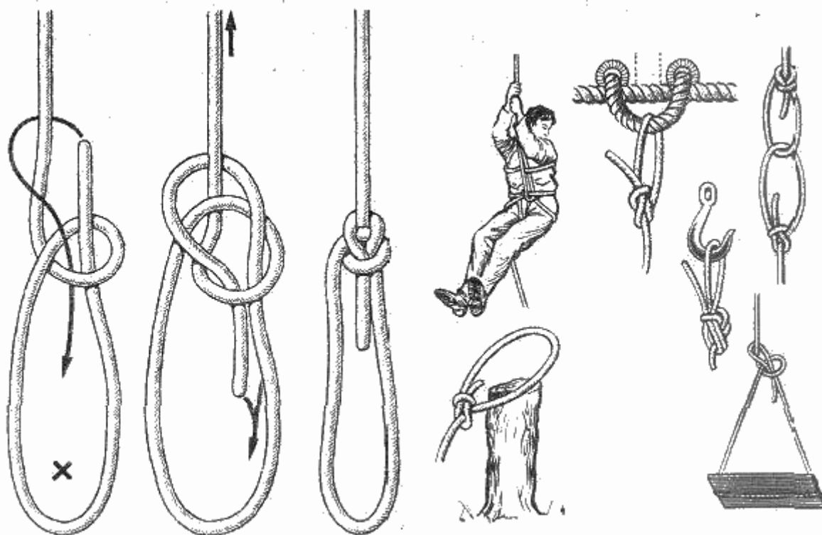
А Рис. 76. Беседочной узел
