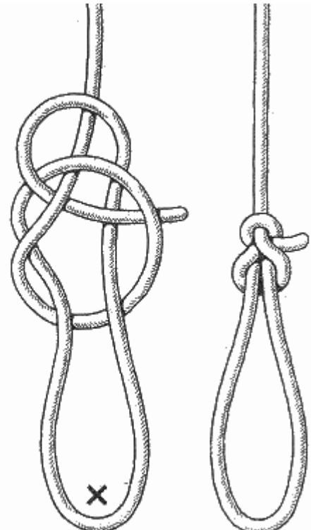
А Рис. 71. Совершенная петля
