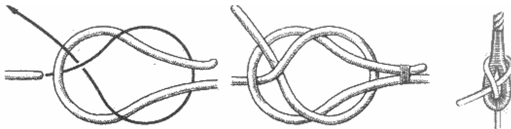
А Рис. 38. Шкотовый узел
