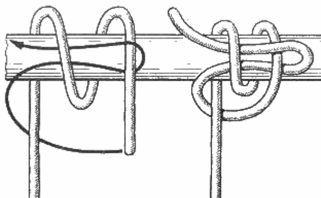
Гис- 56. Лисельный узел
