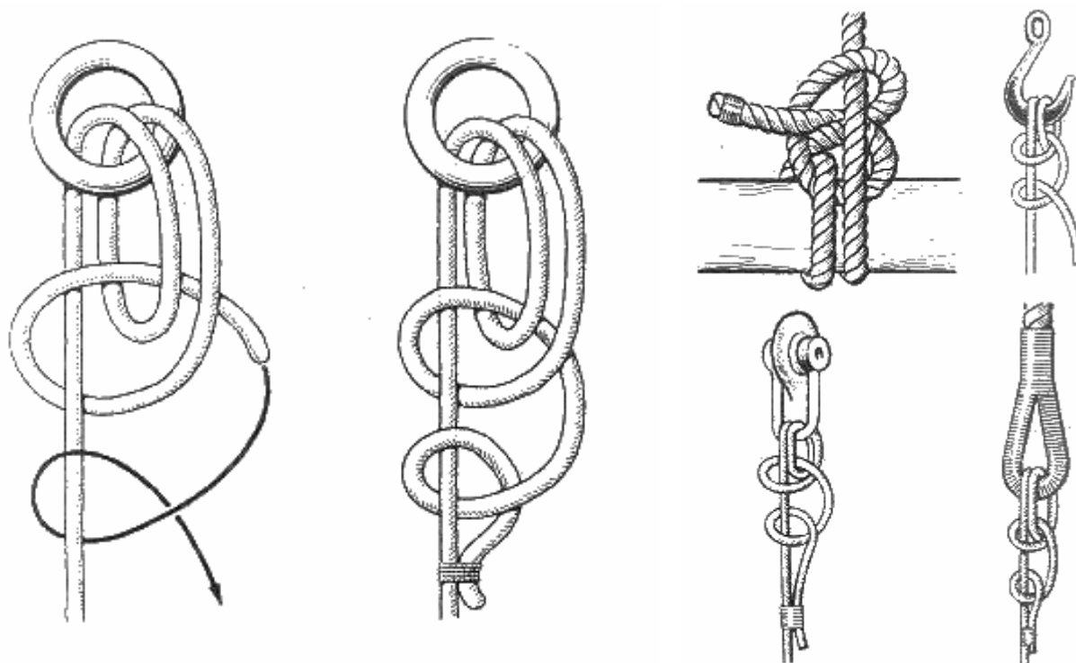
А Рис. 15. Рыбацкий штык (якорный узел)
