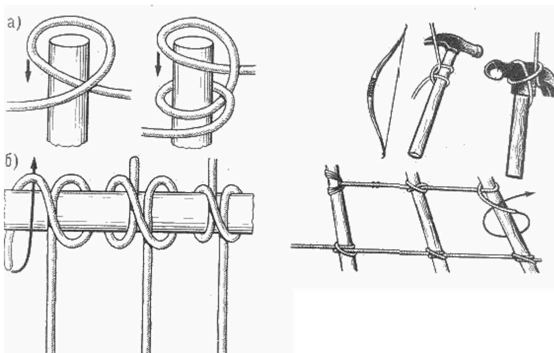
А Рис. 48. Выбленочный узел: а - первый способ вязки; б - второй способ вязки
