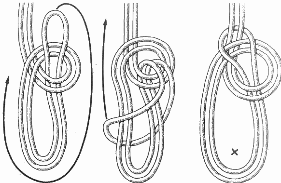
А Рис. 77. Двойной беседочный узел
