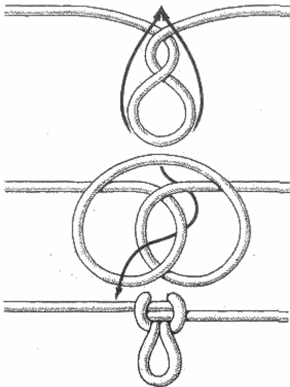
А Рис. 74. Ездовая петля
